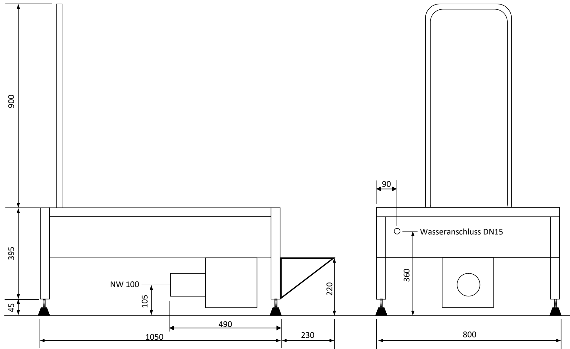
Stiefelwaschanlage STW 337-B Maßdetails
